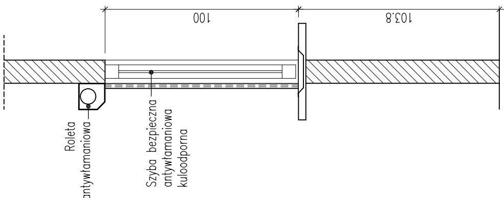
PRZEKRÓJ A-A skala 1:20
